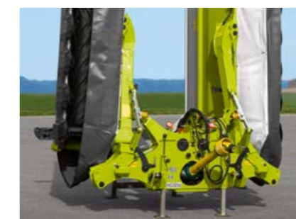
Ahorrando espacio: Estable posición de estacionamiento de todas las macrosegadoras.
